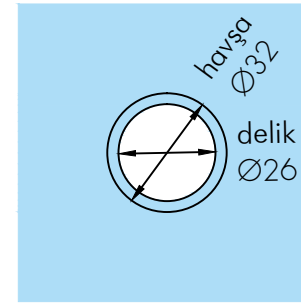
havşalı delik detay
